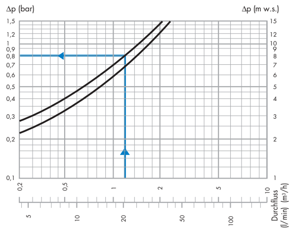
Diagramm 2 (Druckverlust)
